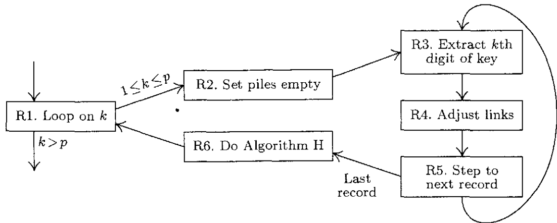
Fig. 32. Radix list sort.
