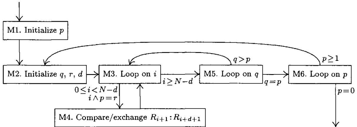
Fig. 17. Algorithm M.
